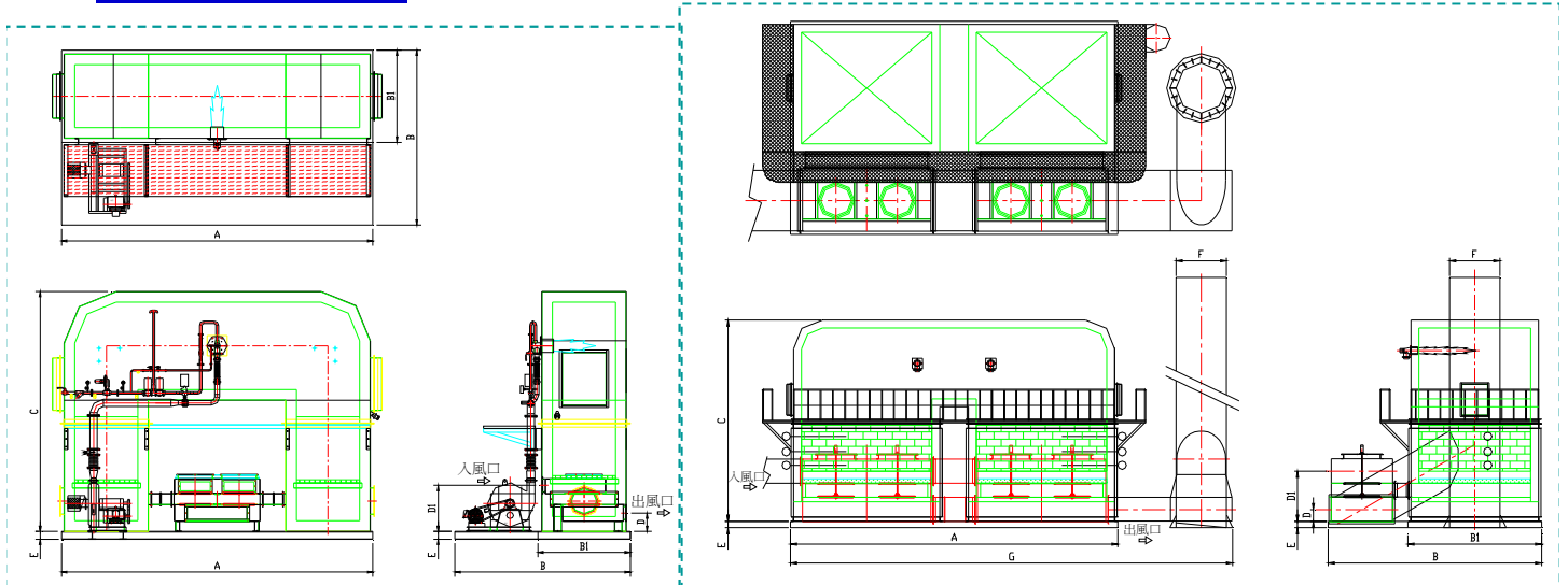
傑智高效能雙槽蓄熱式焚化爐(2T-RTO)尺寸圖
